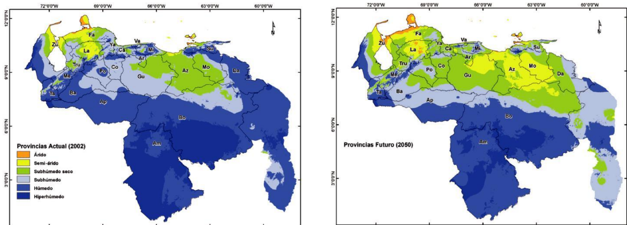
Figura 3. Distribución de las provincias de humedad para los años 2002 y 2050. Las iniciales corresponden al nombre de estados.
